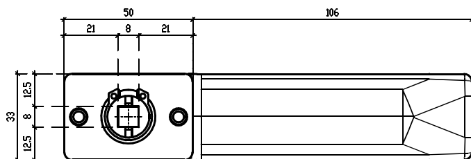
Widok z tyłu klamka I
