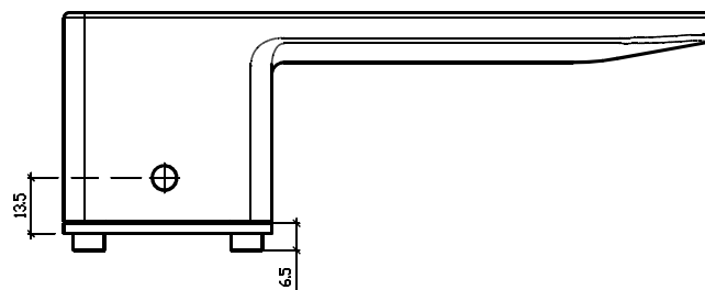
Widok z góry klamka I
