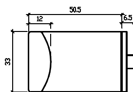
Widok z prawej strony klamka I
